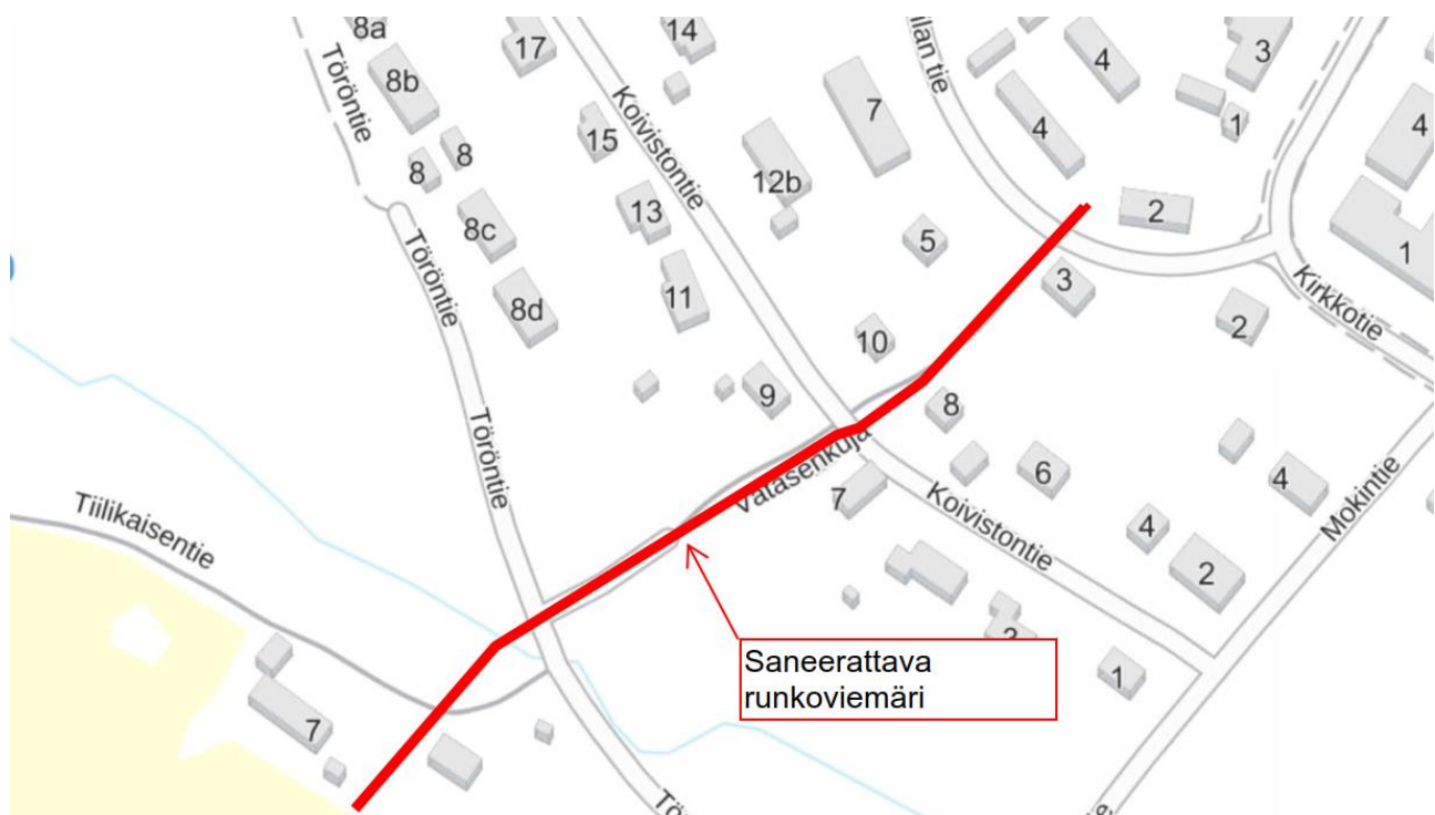
Kuva 1. Saneerattava runkoviemäri
